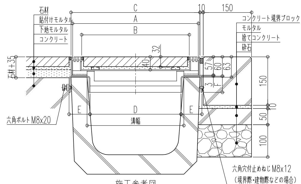
施工参考図
